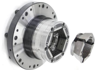
Spannfutter
